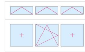
Поворотно-откидное с тремя фрамугами
